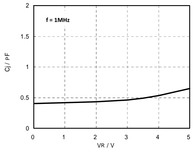
Cj-VR (25°C)
